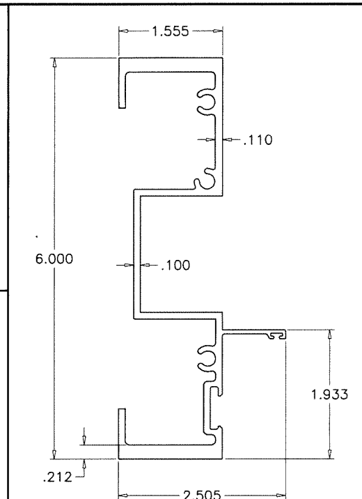
③ FRAME JAMB
